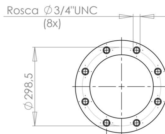
FLANGE TM 8120 E TM 8160
