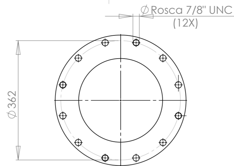
FLANGE TM 8200
