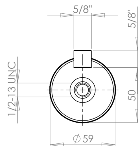
FLANGE TM 8120 E TM 8160
