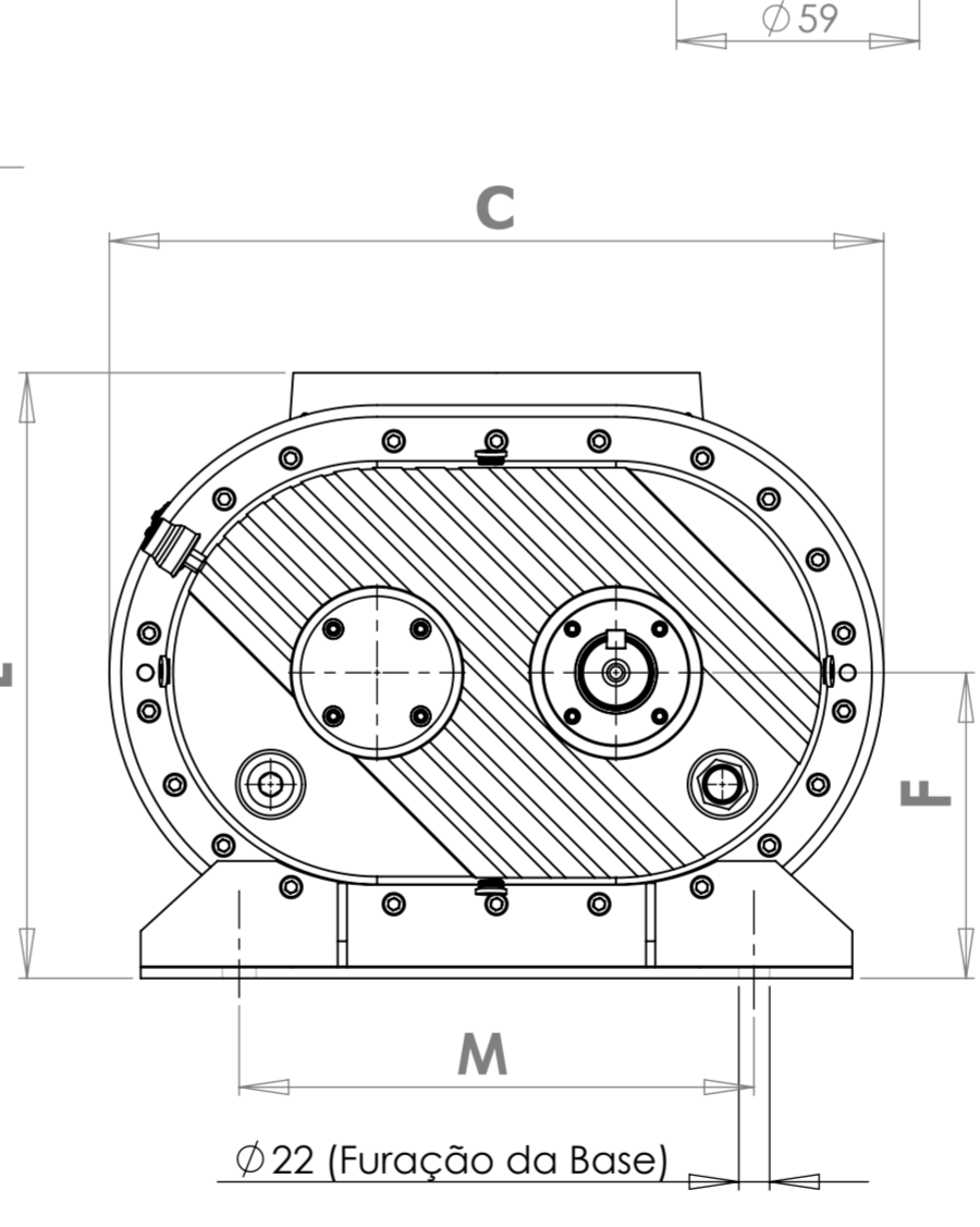
FLANGE TM 8120 E TM 8160
